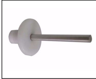
12 No. lu Deneş Sondası (TS EN 61032 Şekil 8)
