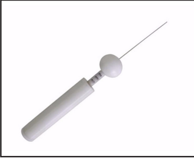
IP4X Test Probu (D Deney Sondası, TS EN 61032 Şekil 4)
