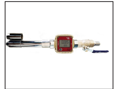
IPX5 ve IPX6 Jet Nozül (Elde taşınabilir)
